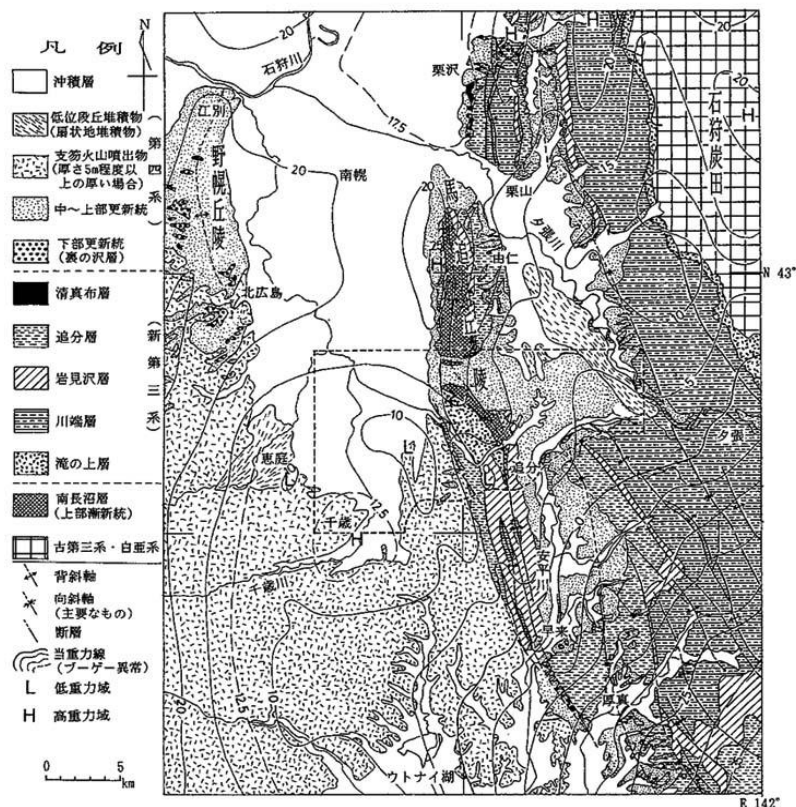
図Ⅲ.1.4-2 馬追丘陵とその周辺の地質概略図（岡，1998より引用） 破線内は千歳地区表層地質報告書の報告範囲。
