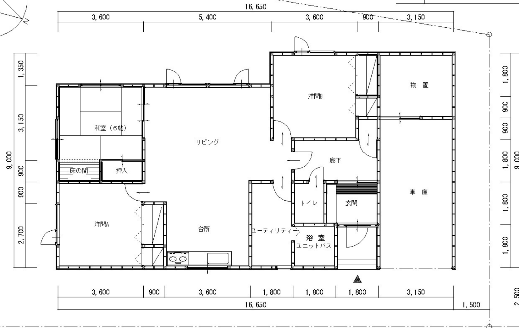
配置図・平面図 S=1:100
