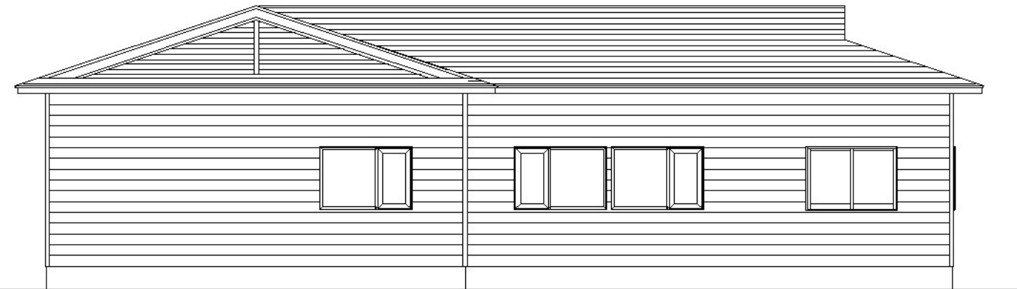
西面立面図
