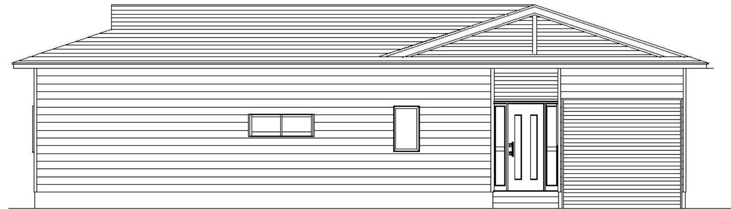
東面立面図
