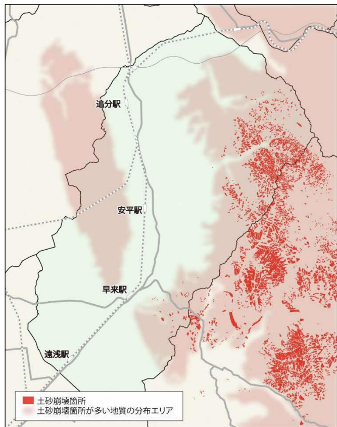
災害での土砂崩壊地点と地層分布
