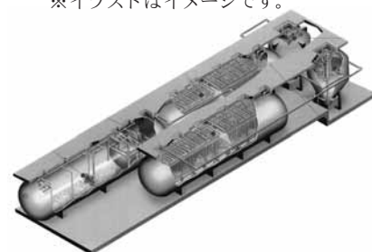
工場製作型極小規模処理施設 ※イラストはイメージです。
