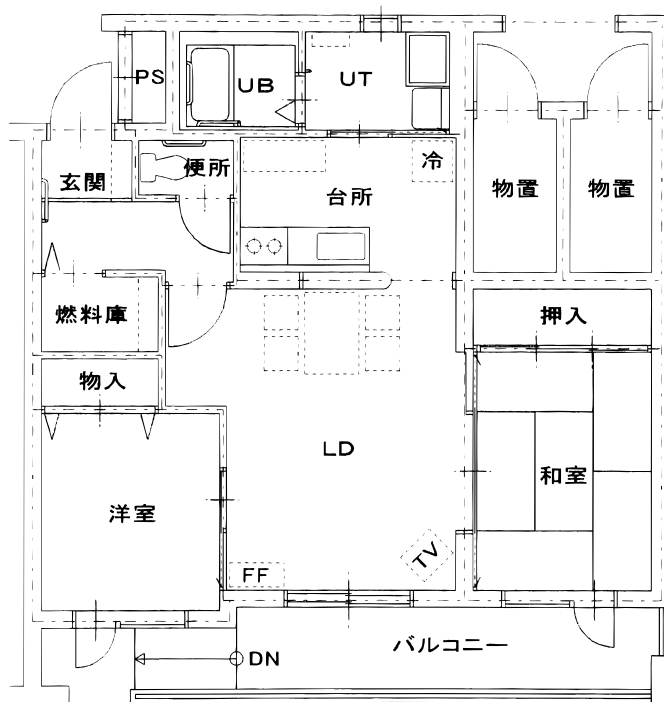
C1タイプ 1階 2LDK (21坪) 1戸
